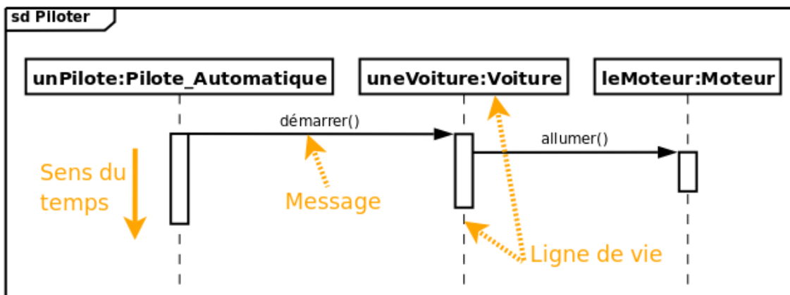
Figure 7.5 : Diagramme de séquence d'un système de pilotage.
