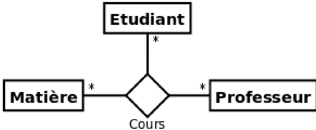
Figure 3.6 : Exemple d'association n-aire.
